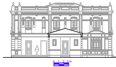
Elevation 02
